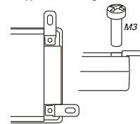
Montaje en tapa Upper lid mounting
