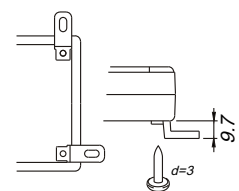
Montaje en base Bottom lid mounting
